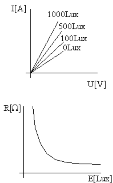
VA charakteristika
